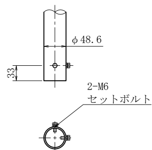
適合アーム参考図
