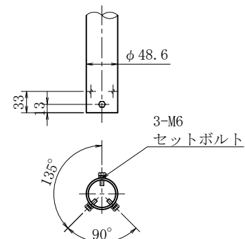
適合アーム参考図
