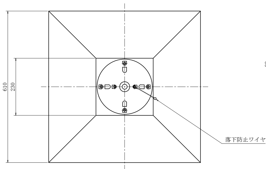
適合アーム参考図
