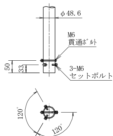
適合アーム参考図
