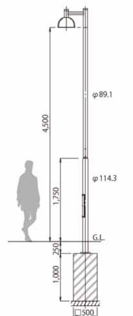
基礎図は、標準的な地盤のときの参考です。
